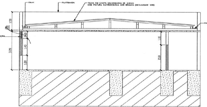
CORTE A-B ESCALA = 1:50
